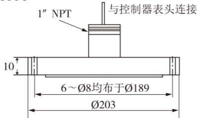
平板探头L890C
