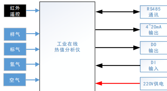
热值仪在应用系统中的接口示意图
