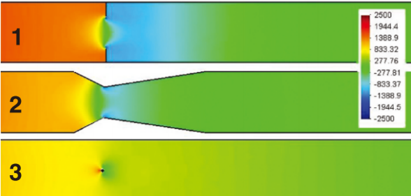
三种压损比较: (1)孔板; (2)文丘里管; (3)德尔塔巴探头
