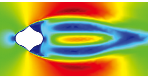
流速变化色谱，整流加速段将流速加速3倍
