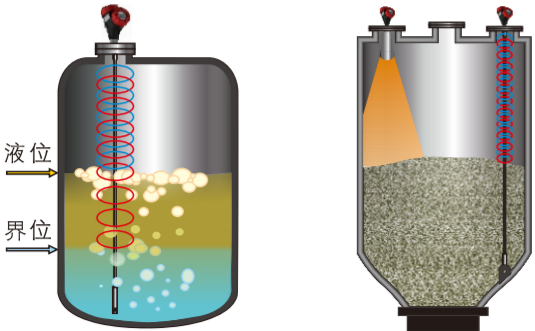
发射的雷达波有较强的穿透力，配合特殊的算法，能实现界液位的测量。 由于雷达波所具有的穿透特性，同样适用于大量程，多粉尘的固体场合。
